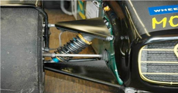
Figur 1 Viser bærearms vinger for biler med klassisk karosseri iht. Pkt. 238.3.4 i Teknisk reglement for Super Seven Racing.
