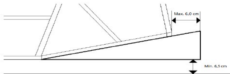
Figur 4 Viser en tegning af den alternative diffusor. Materiale frit og maksimal bredde på 113.0cm og kun en på hver side. Iht. pkt. 238.3.4 i Teknisk reglement for Super Seven Racing.
